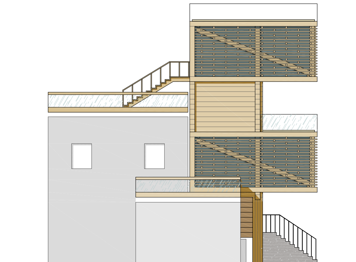
Южный фасад
