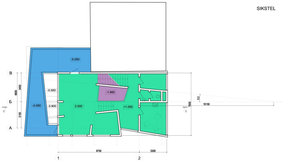
ARTPLAY ДОМ НА КРЫШЕ Лист 3. План на уровне 1 этажа Отм. 0.000, +1.050 М 1:100
