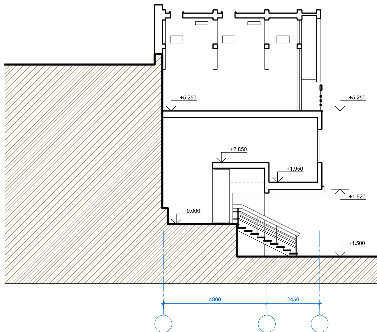
РАЗРЕЗ 1-1
