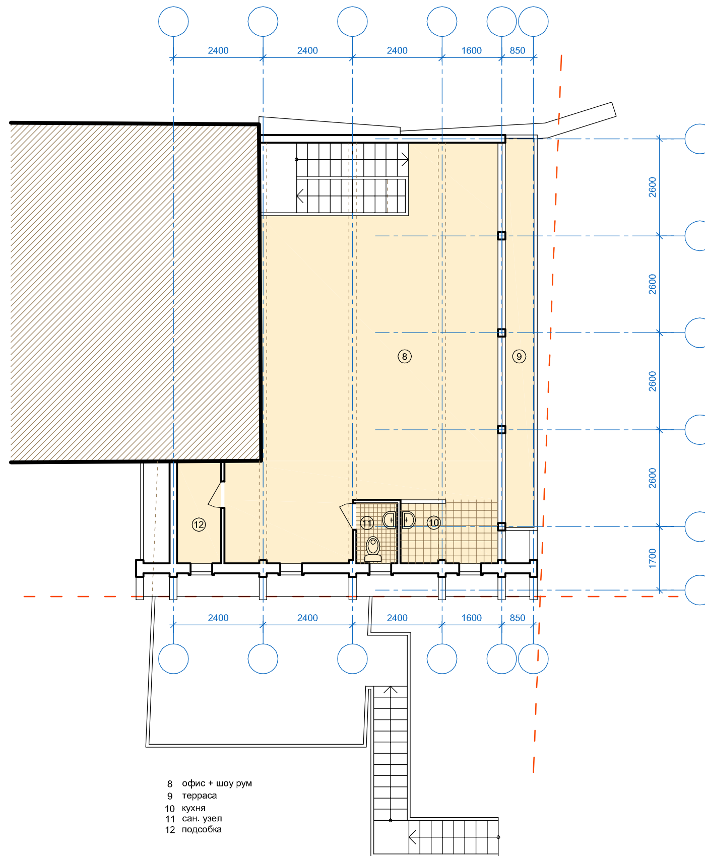
ПЛАН 2 ЭТАЖА
