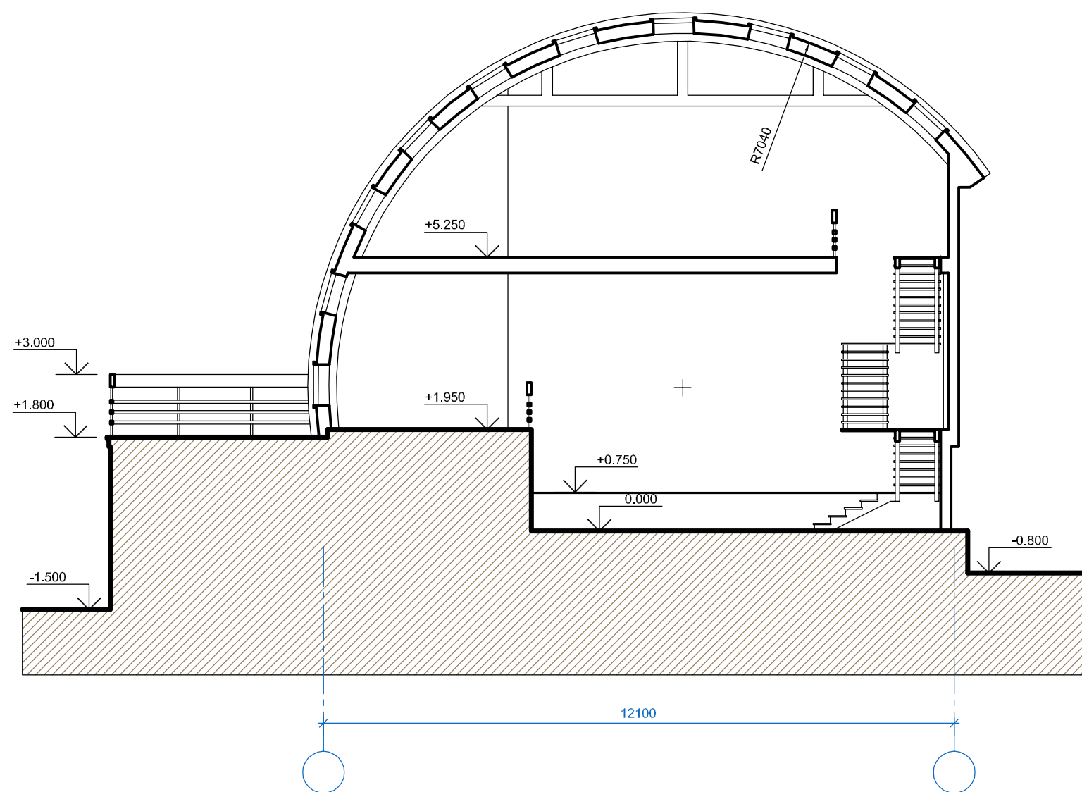
РАЗРЕЗ 2-2
