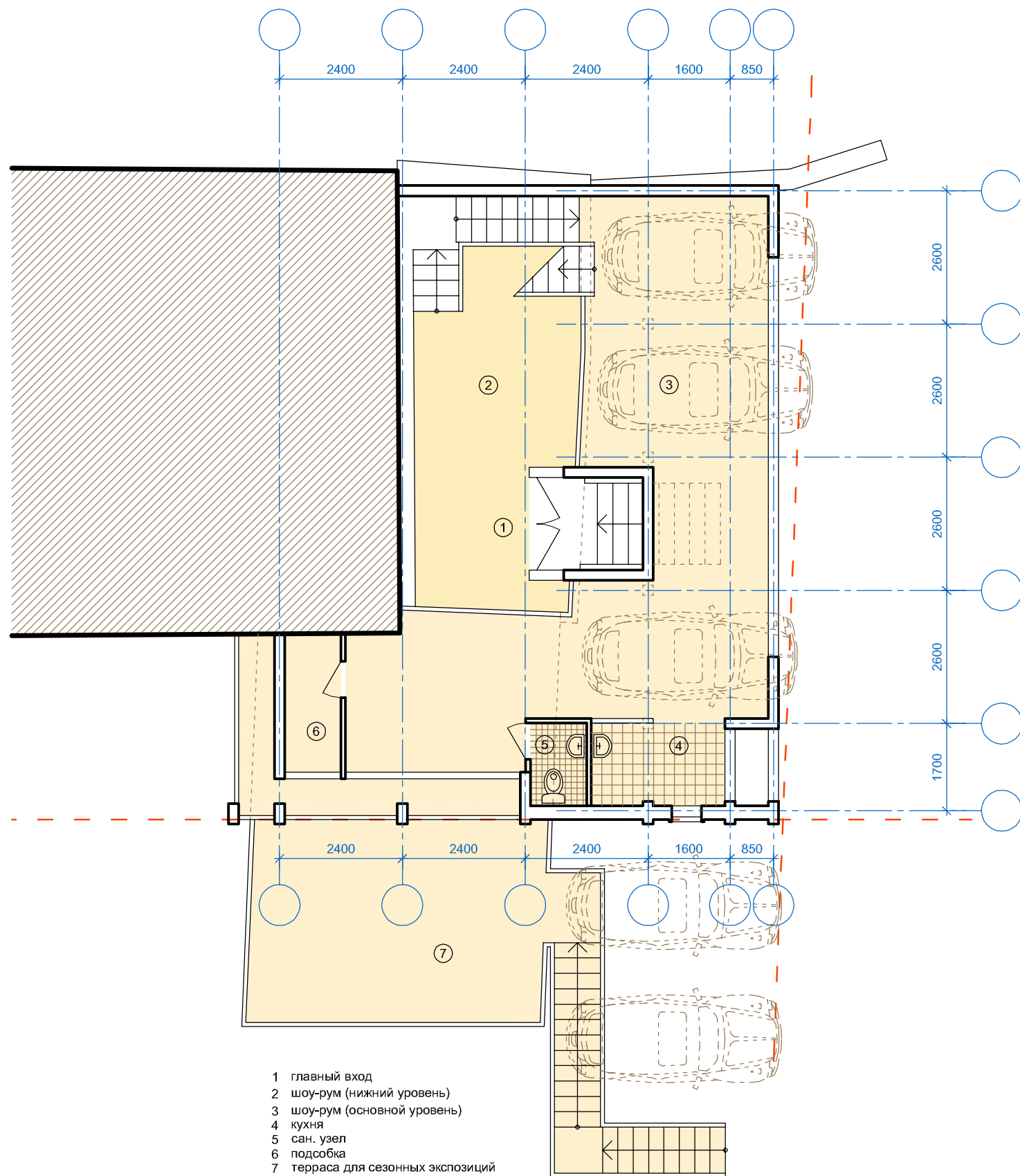
ПЛАН 1 ЭТАЖА
