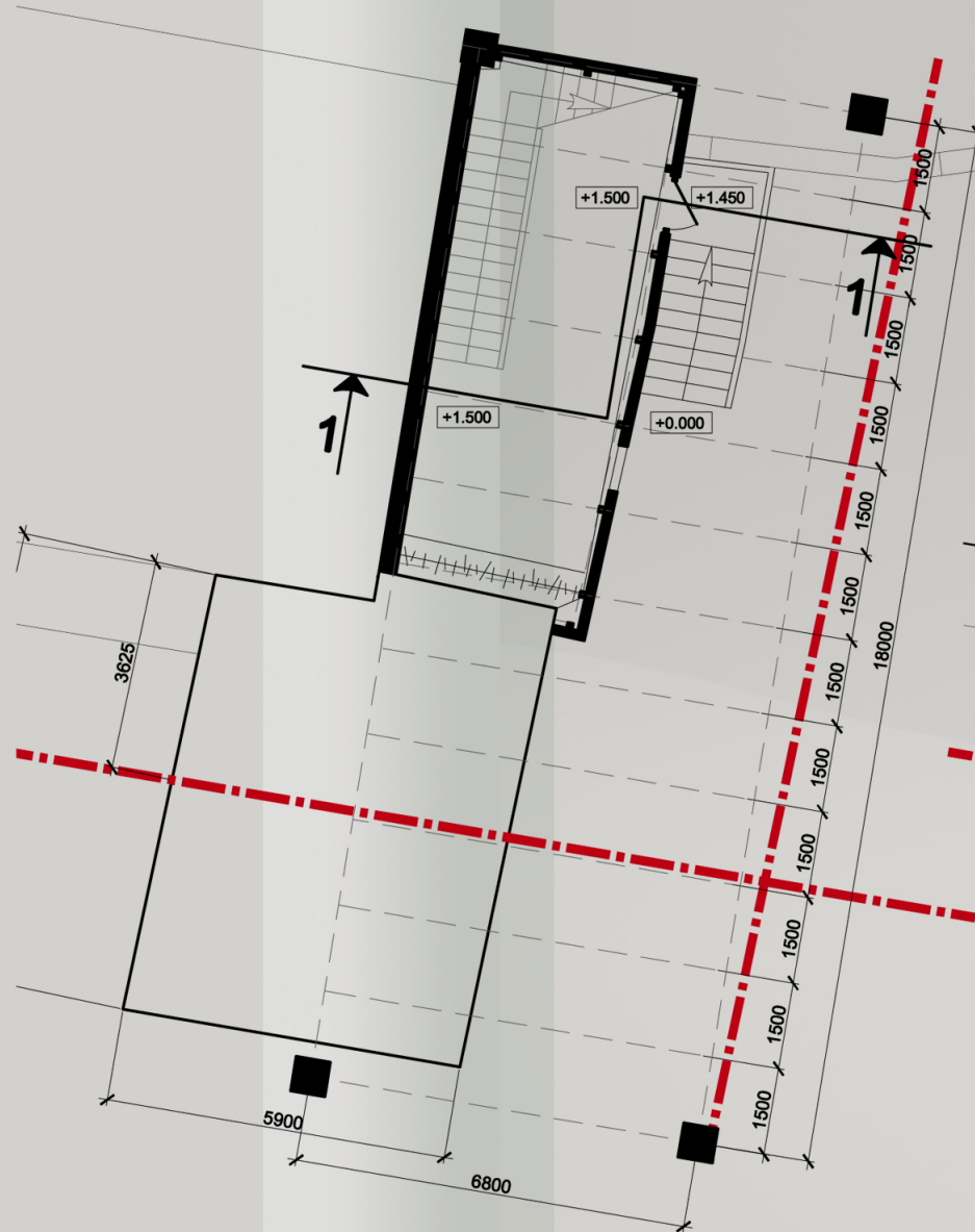
План 0-го этажа (М 1:100)
