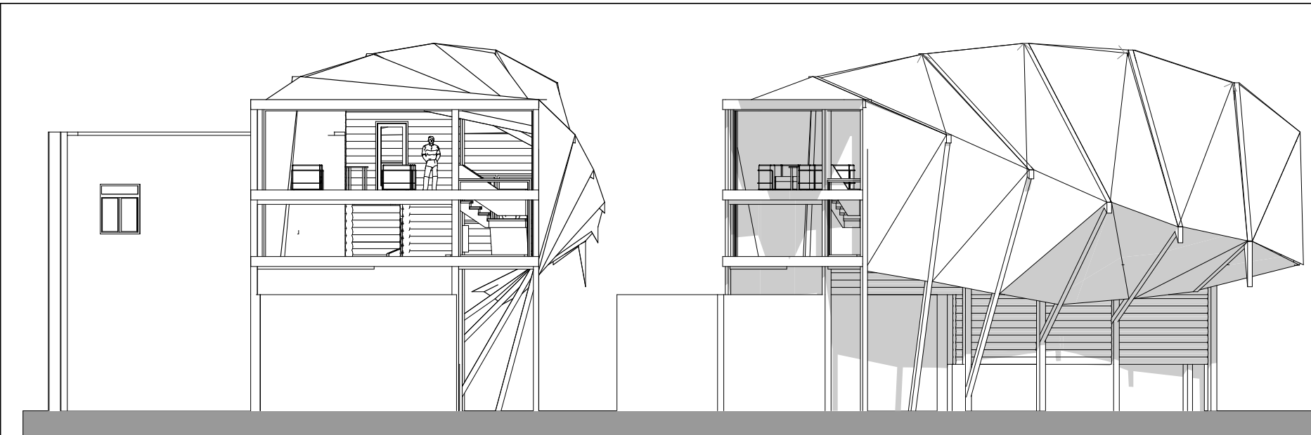
Фасады М 1 100
