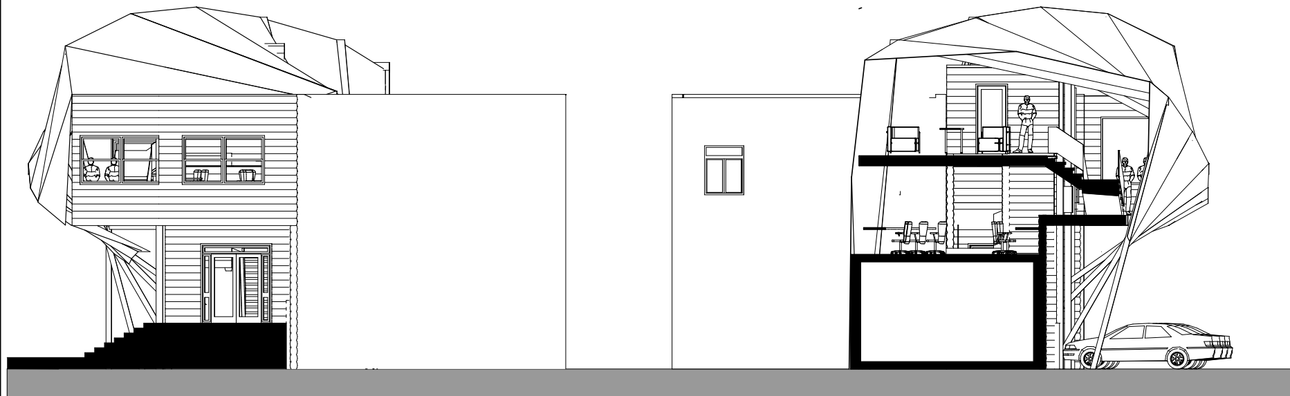
Фасады М 1 100
